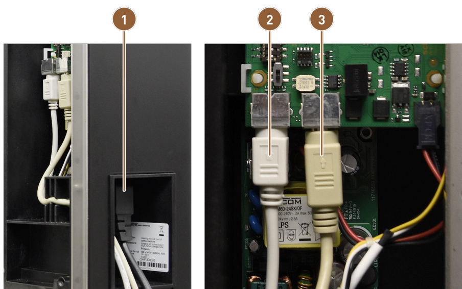
Abb.: ProCare-Kabelanschlüsse
