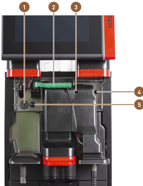
Abb.: Bedienelemente in der Maschine
