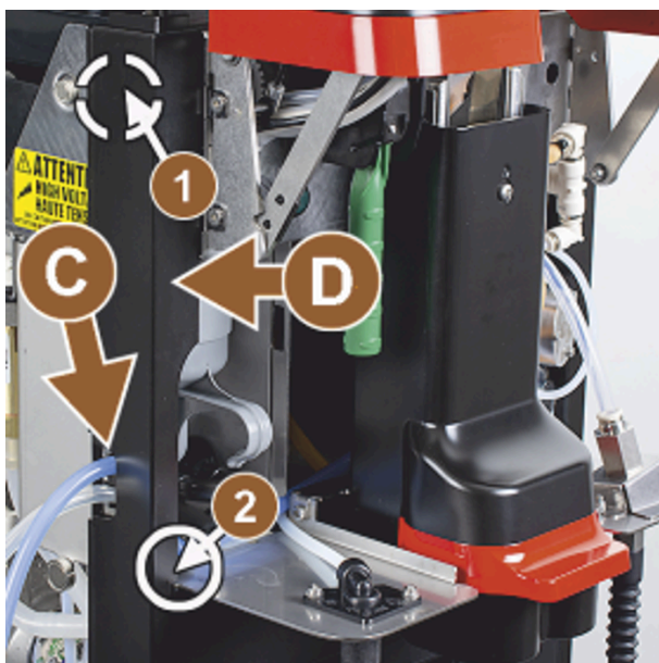
Abb.: Milchschräuche durch Seitenleiste
