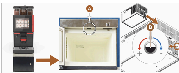
Abb.: Unterstellkühleinheit einschalten und einstellen
