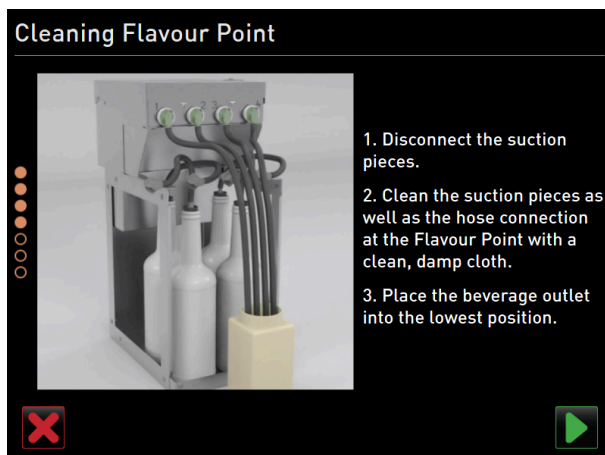
Abb.: Reinigungsbehälter an Flavour Point anschliessen
