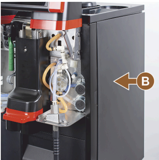
Abb.: Montage der rechten Seitenverschalung
