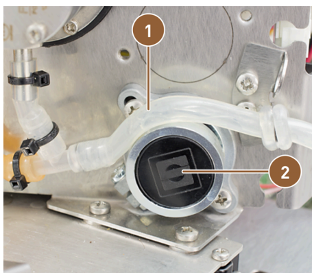
Abb.: Milchschläuche in Quetschventile einsetzen (Twin Milk)
