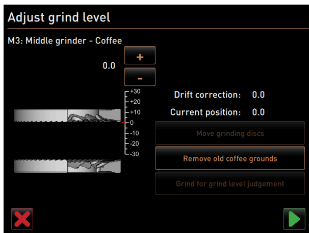
Abb.: Mühle anpassen: altes Kaffeemehl entfernen
