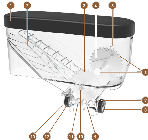
Abb.: Teile des Standard-Pulverbehälters (2 kg)
