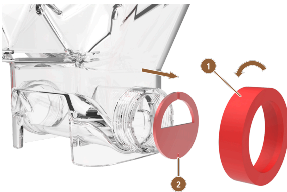
Abb.: Standard-Pulverbehälter: Dosierelemente entfernen
