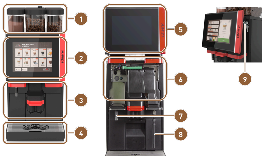
Abb.: Maschinenübersicht
