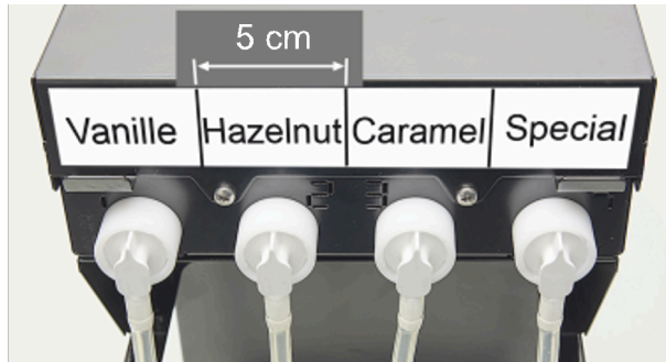
Abb.: Beschriftungsbeispiel für Schlauchanschlüsse Sirupflasche zu Siruppumpe
