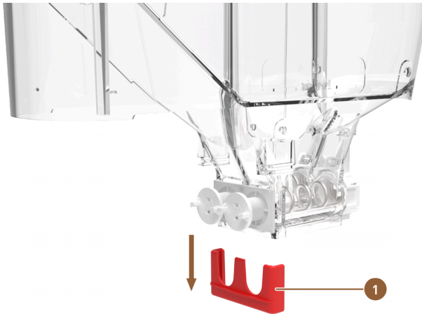
Abb.: Twin-Pulverbehälter: Antriebshalterung entfernen
