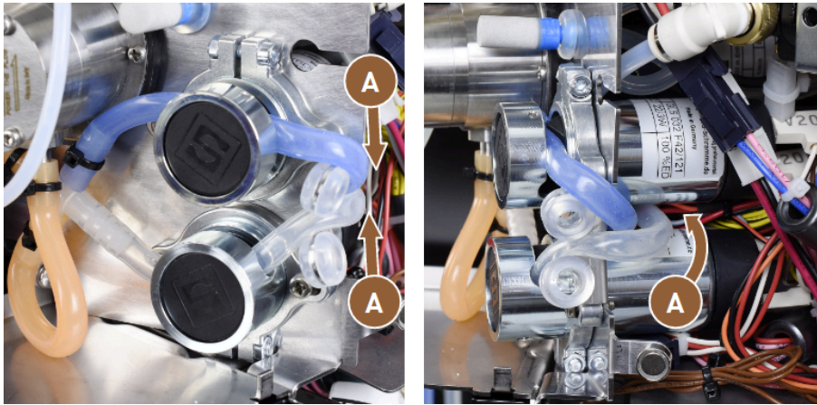
Abb.: Milchschräume verlegen
