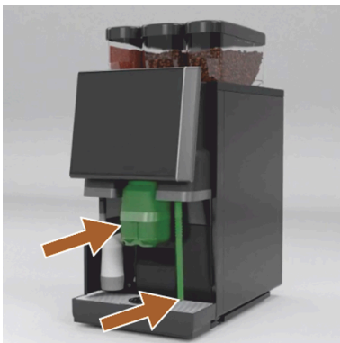
Abb.: Tassenrost entfernen
