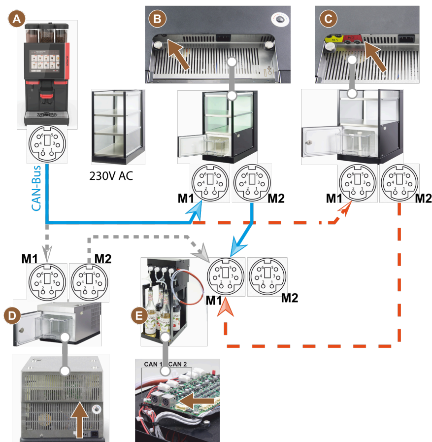
Abb.: CAN-Bus-Verbindungen von der Maschine zu Beistellgeräten (Beispieldarstellung)
