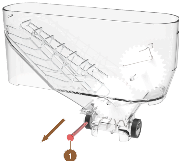
Abb.: Standard-Pulverbehälter: untere Achse entfernen
