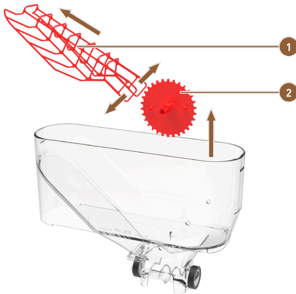
Abb.: Standard-Pulverbehälter: Pulverschaufel entfernen
