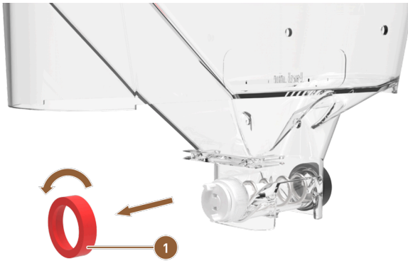
Abb.: Standard-Pulverbehälter: Überwurfmutter an Förderseite entfernen
