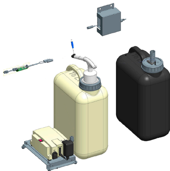
Abb.: Externer Trink- und Schmutzwassertank
