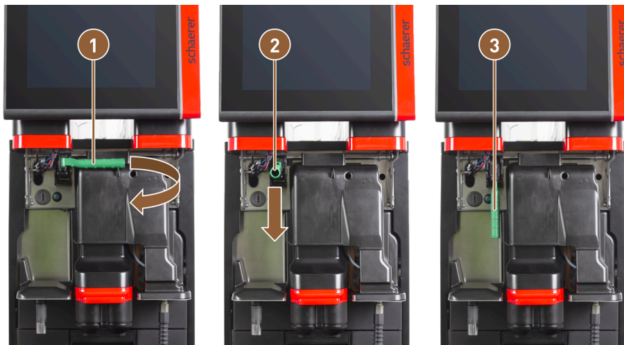
Abb.: Entriegelung Bohnenbehälter und Pulverbehälter (Option)
