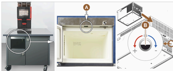
Abb.: Unterthekenkühleinheit einschalten und einstellen
