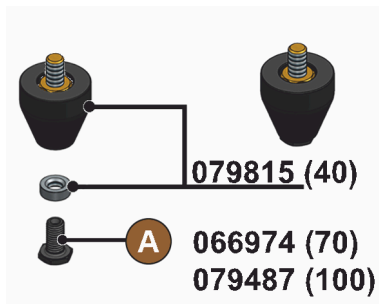
Abb.: Fuss 40/70/100 mm (Lieferung ohne Schraube [A])
