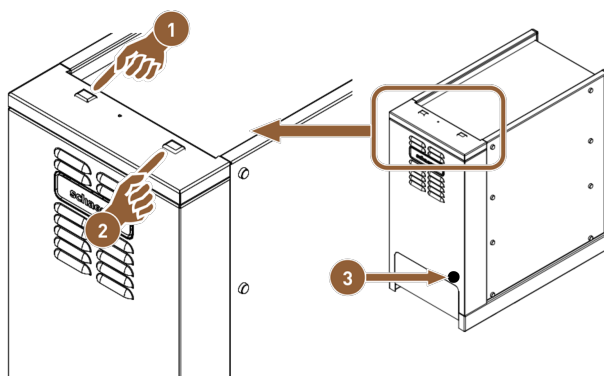
Abb.: Bedienelemente Cup & Cool, Tassenwärmer
