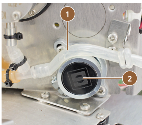
Abb.: Milchschauch in Quetschventil einsetzen (Single Milk)
