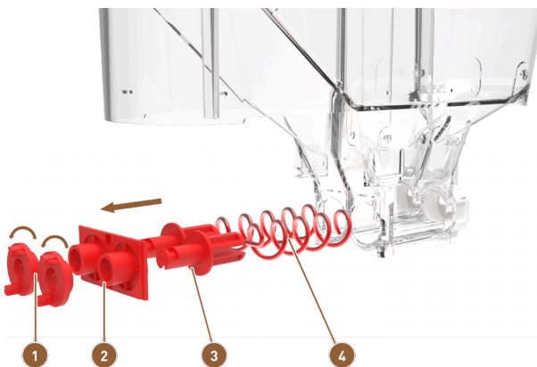
Abb.: Twin-Pulverbehälter: Fördereinheit zerlegen
