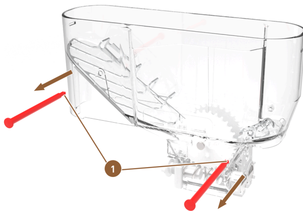
Abb.: Twin-Pulverbehälter: Querstreben entfernen
