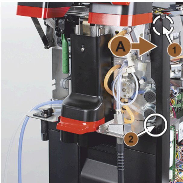
Abb.: Montage der rechten Seitenleiste
